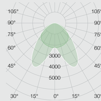
OfficeLUX RAYET 2.0 doppelt asymmetrisch
