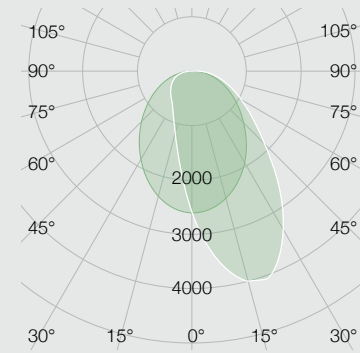
OfficeLUX RAYET 2.0 asymmetrisch
